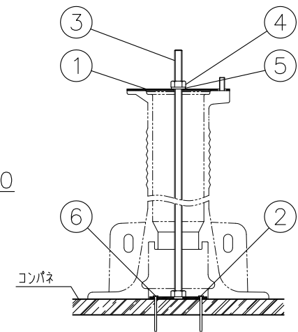
打込金具 設置図
