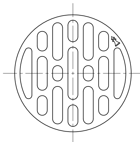
MODEL : ロック式ストレーナ \phi 76
