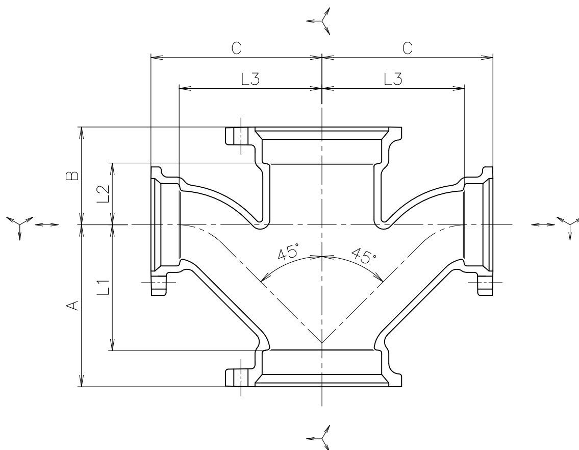
継手各部の名称
