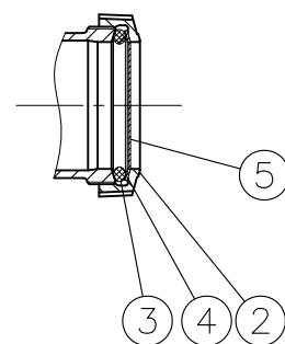
出荷時の部品構成
