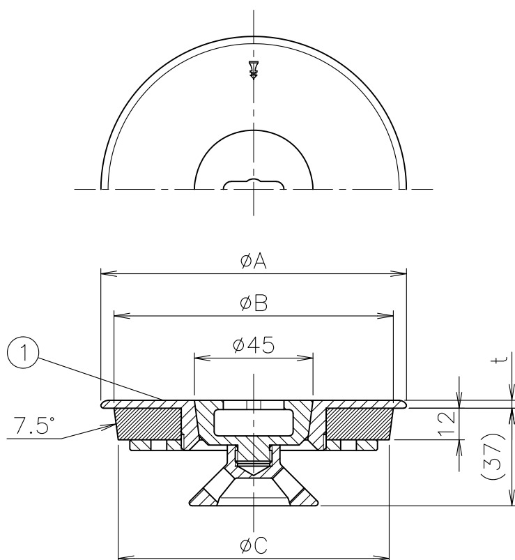
寸法表
