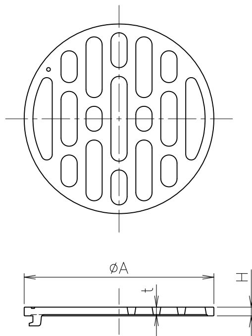
MODEL : ロック式ストレーナ \phi 76
