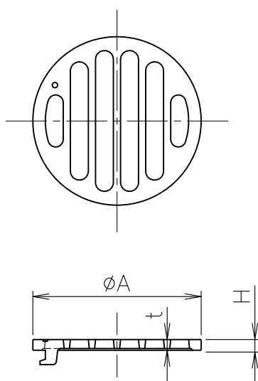
MODEL : ロック式ストレーナ \phi 47
