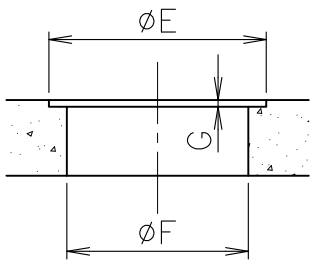
取付け穴寸法
