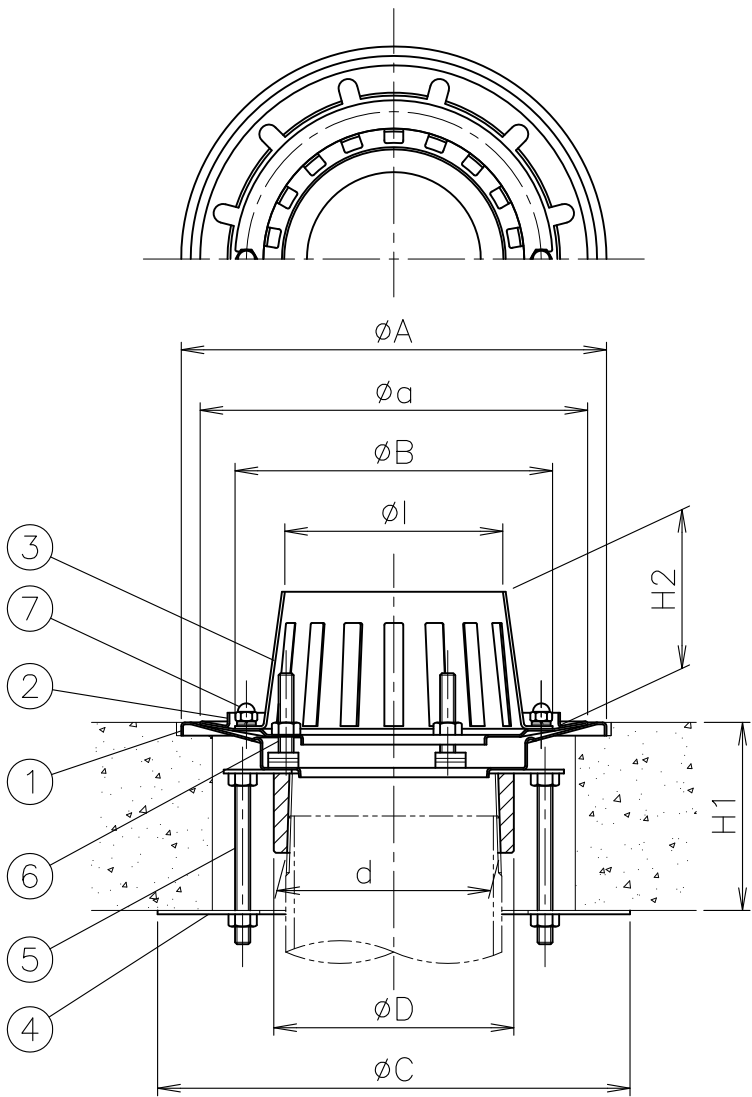
寸法表 単位:mm
