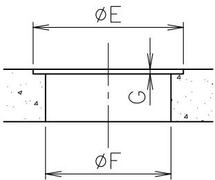
取付け穴寸法
