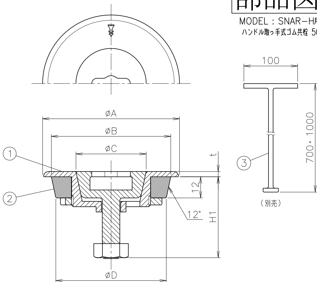
寸法表
