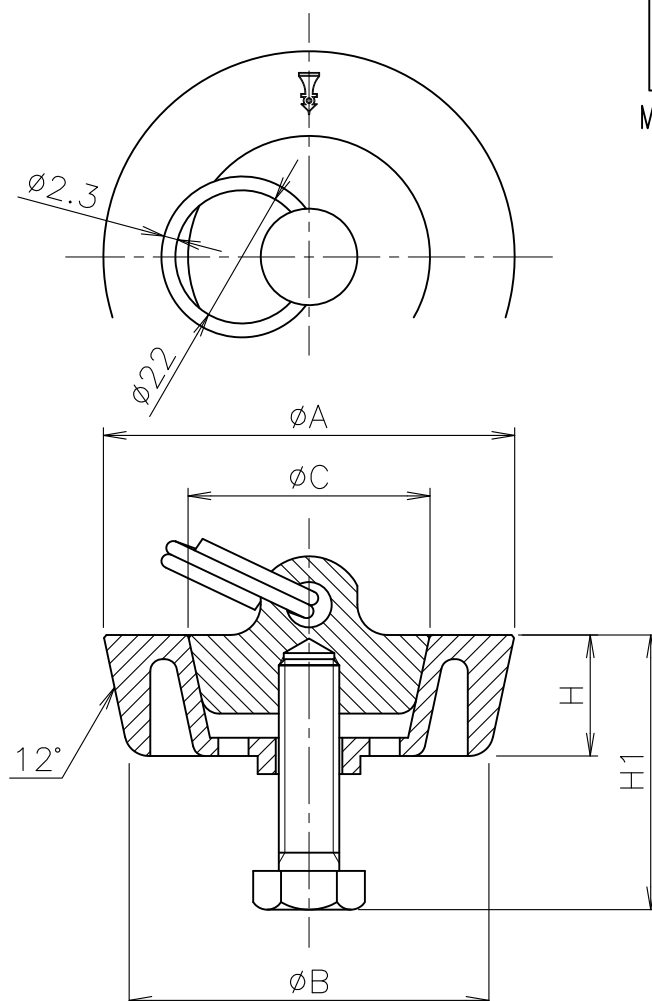
寸法表
