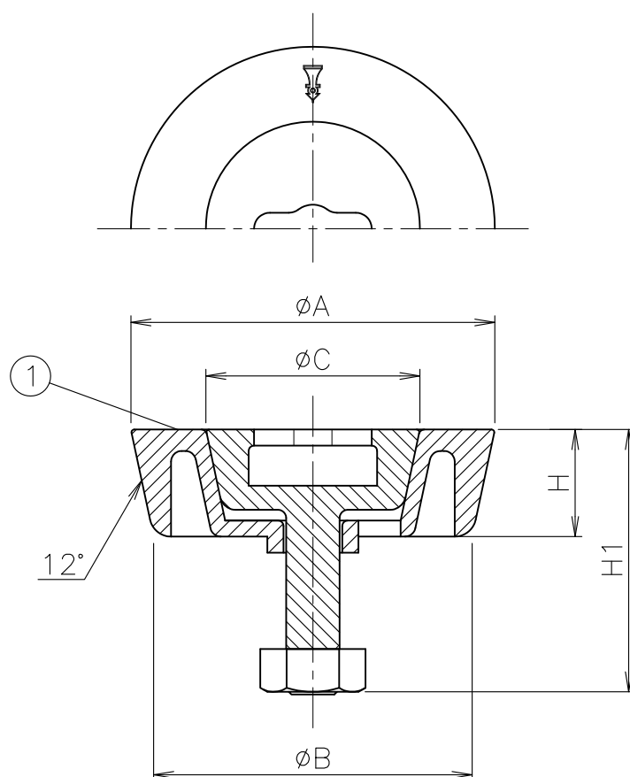
寸法表
