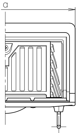
打込金具 固定図(1:2)
