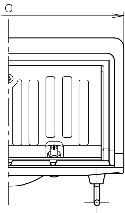
打込金具 固定図(1:2)
