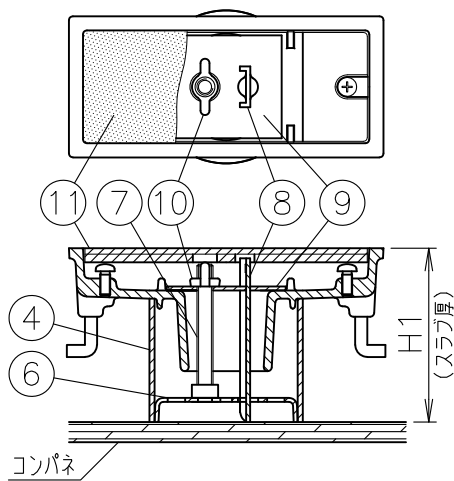
打込金具 固定図(2:3)
