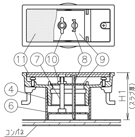
打込金具 固定図(2:3)
