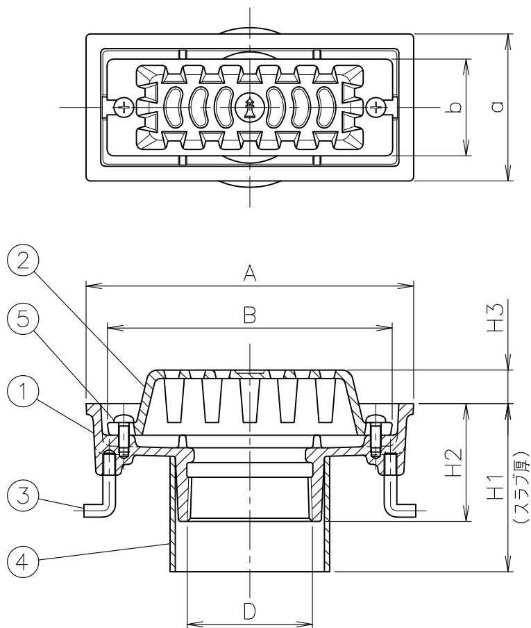
寸法表
