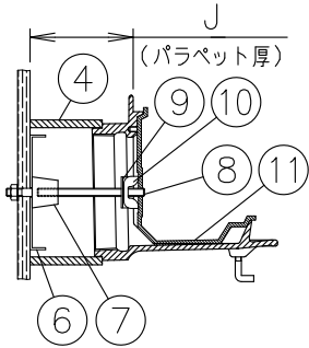
打込金具 固定図(1:2)
