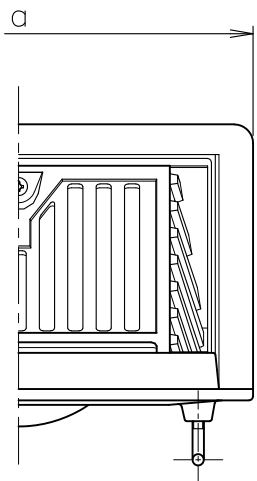
打込金具 固定図(1:2)
