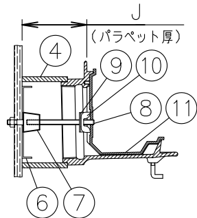
打込金具 固定図(1:2)
