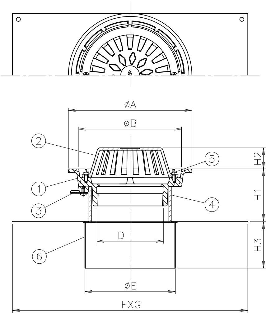
寸法表 単位:mm
