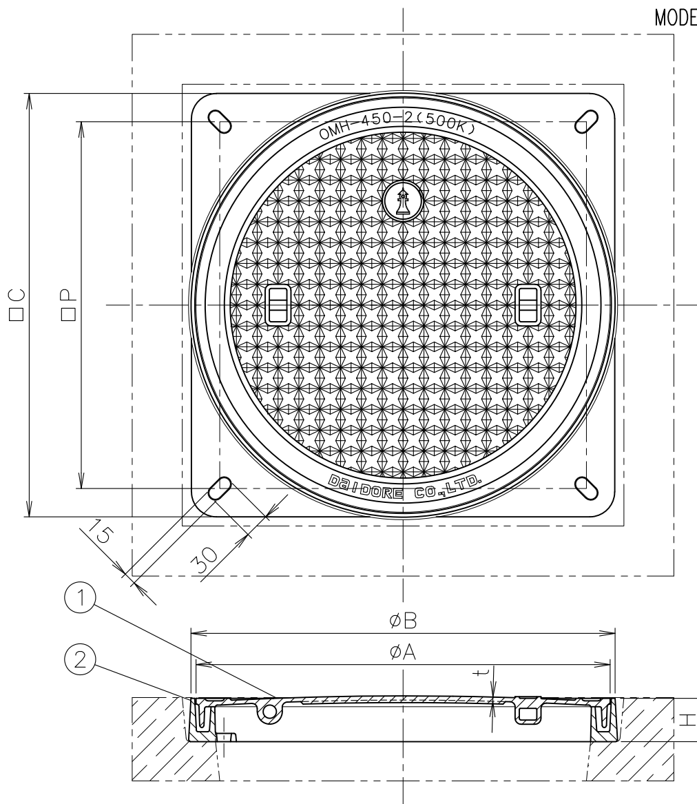
寸法表
