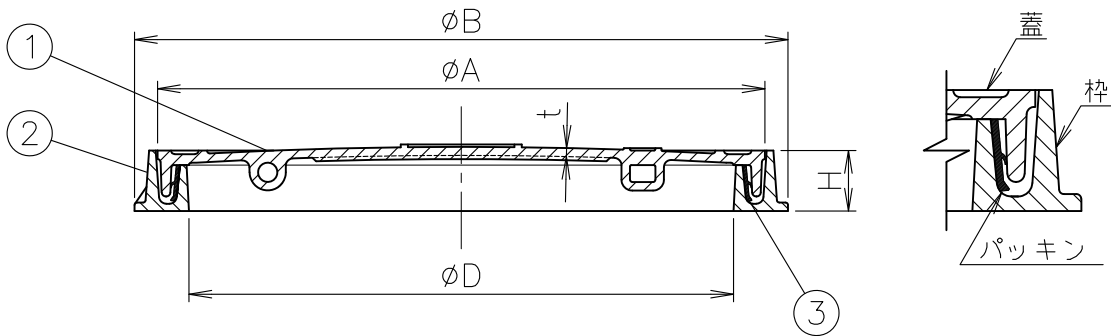
端部詳細
