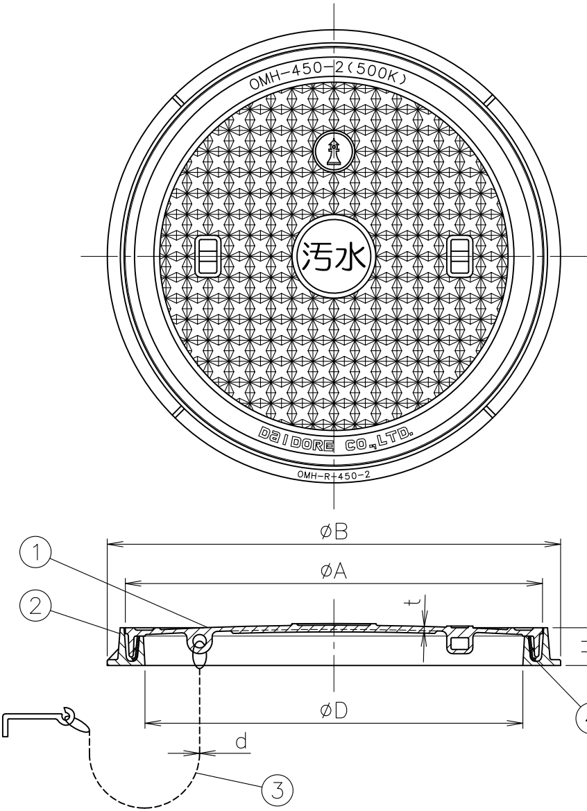
端部詳細
