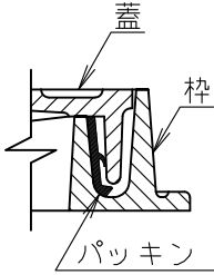
端部詳細
