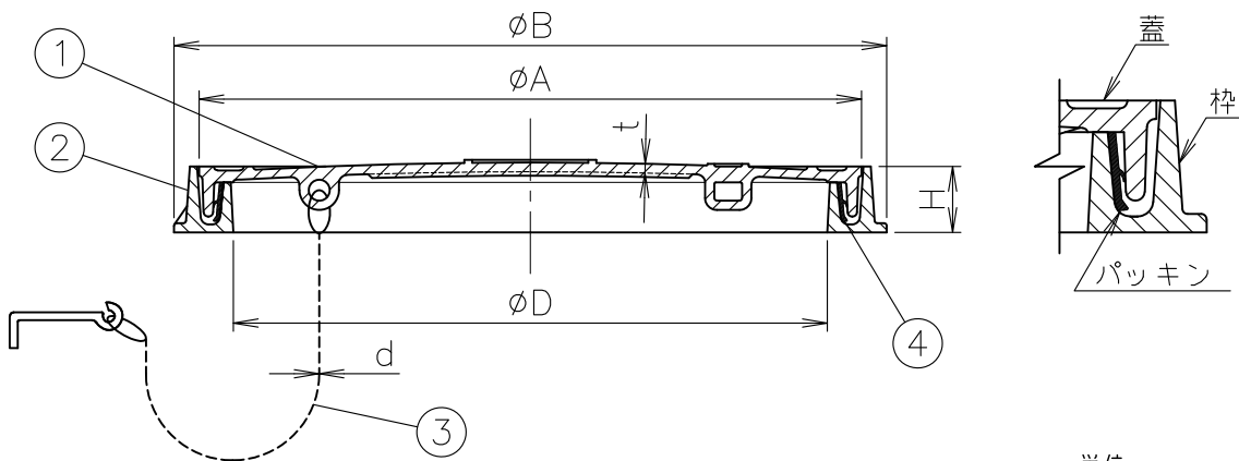
端部詳細
