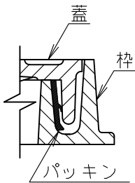
端部詳細
