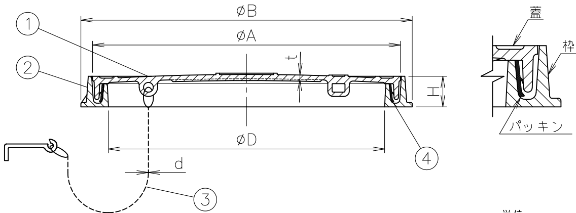
端部詳細
