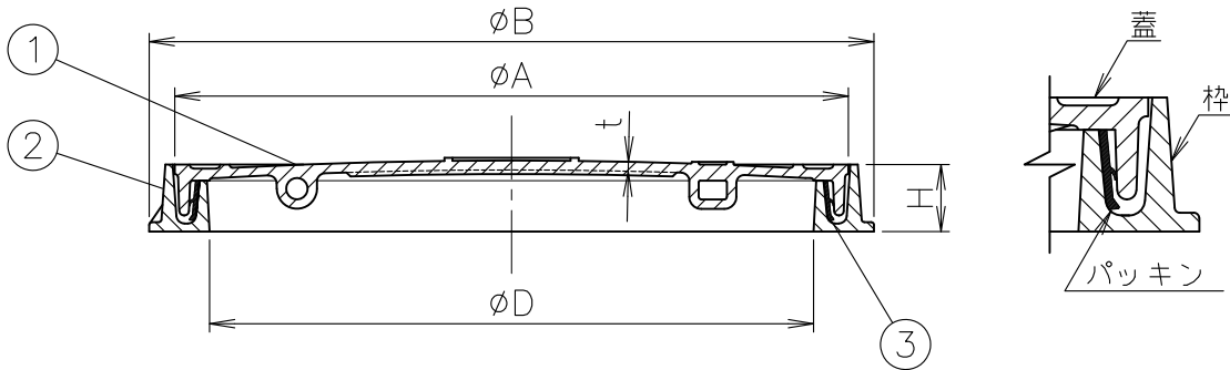
端部詳細
