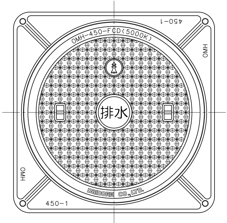
端部詳細
