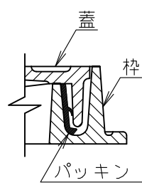
端部詳細
