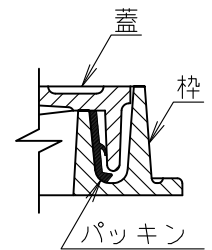
端部詳細
