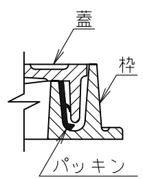
端部詳細
