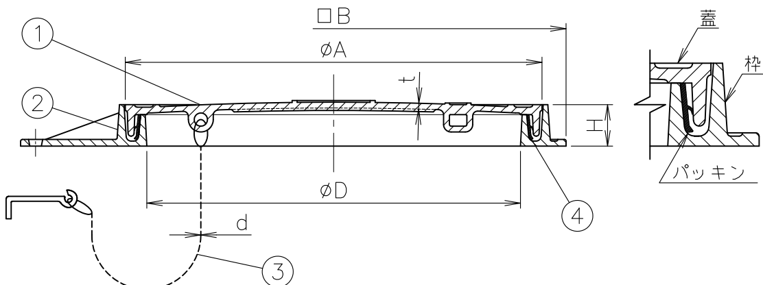
端部詳細
