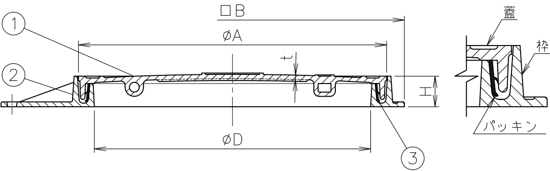
端部詳細
