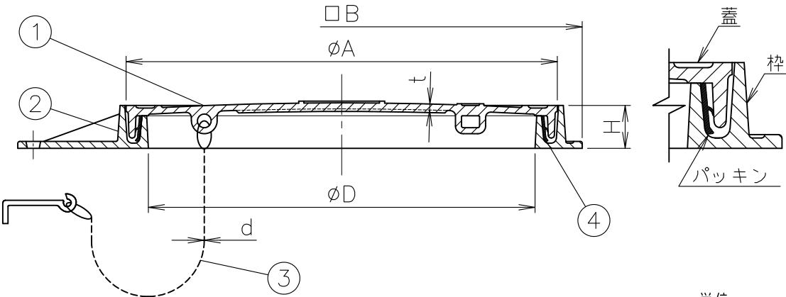
端部詳細
