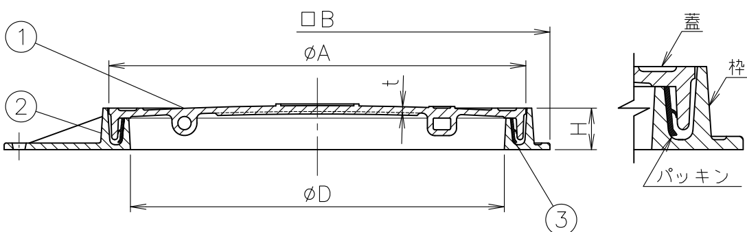
端部詳細
