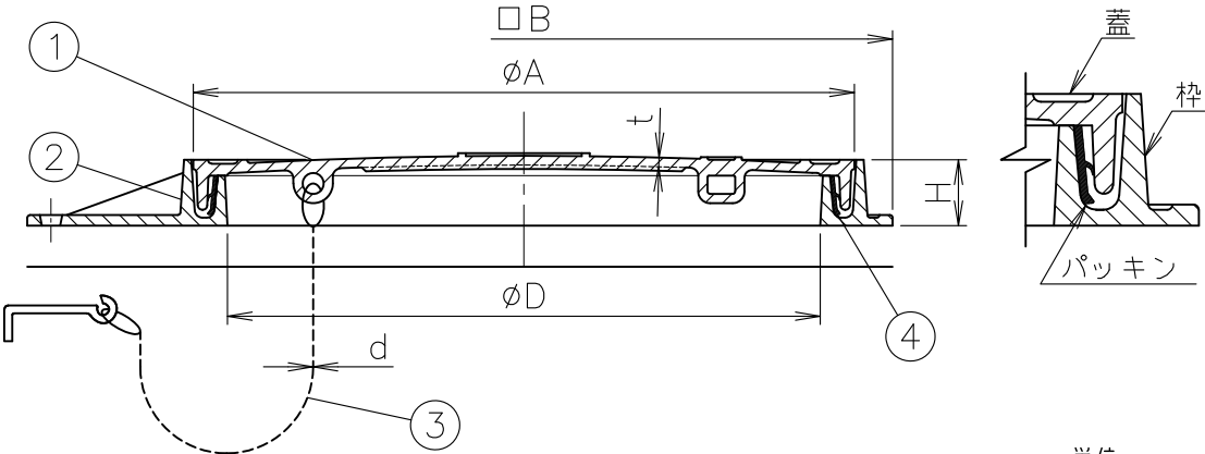
端部詳細
