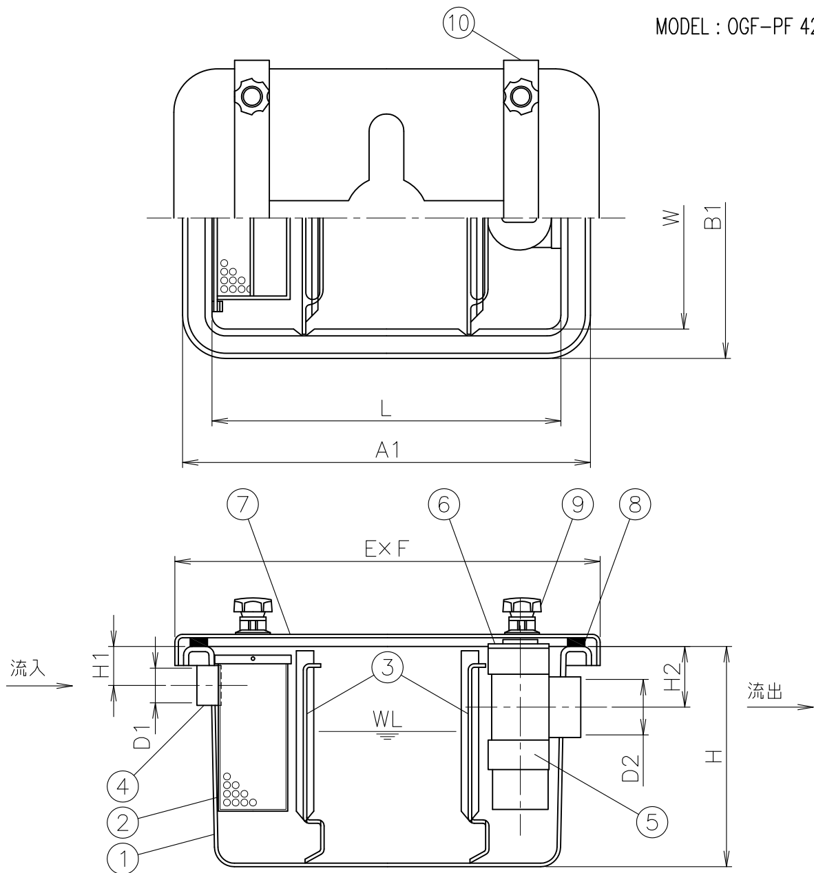
寸法表
