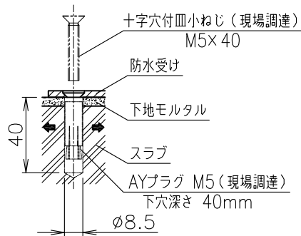
アンカー施工例
