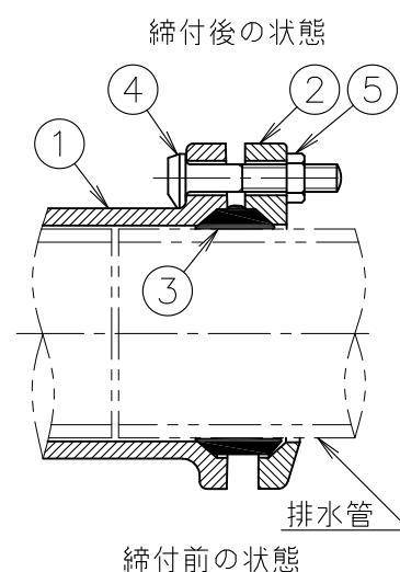
継手各部の名称
