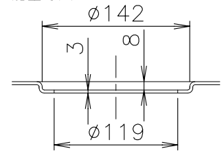
防水パン取付 加工寸法
