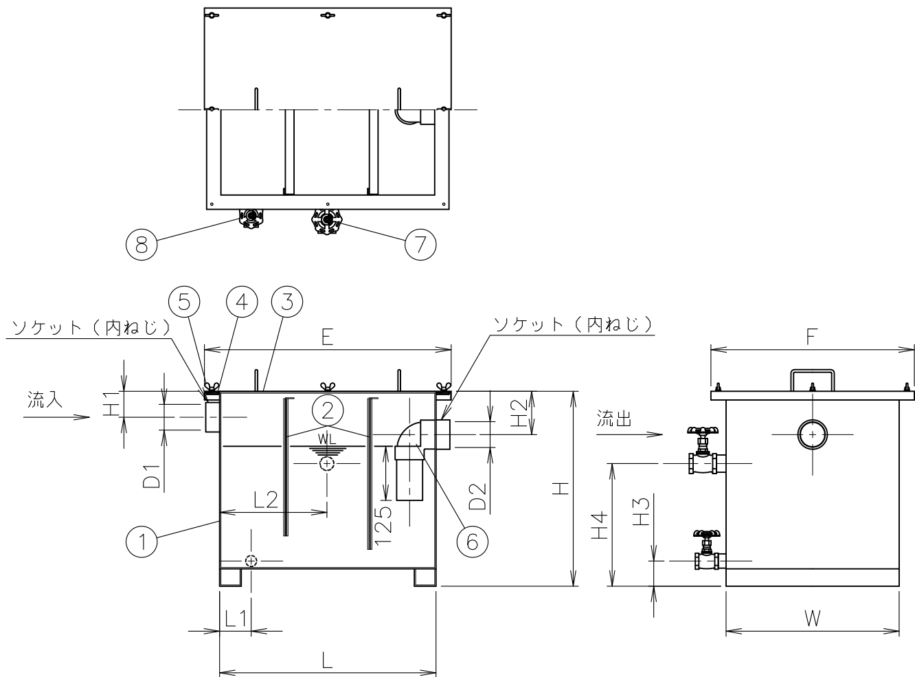
寸法表
