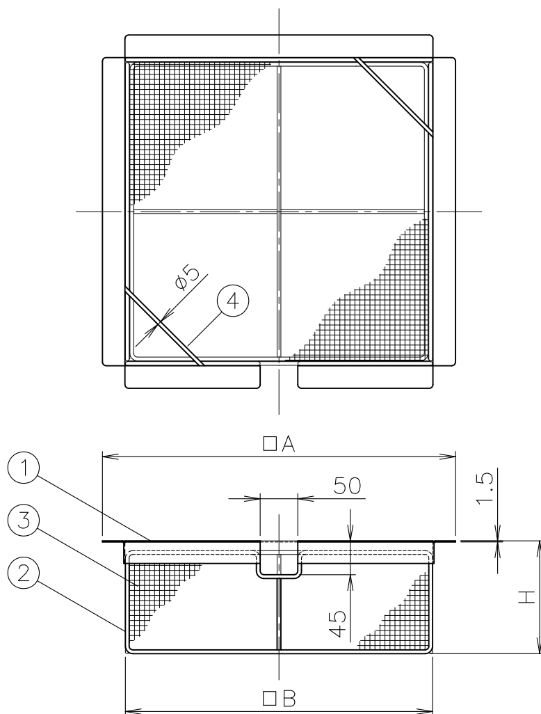
寸法表
