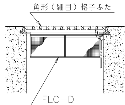
施工例(1:2)
