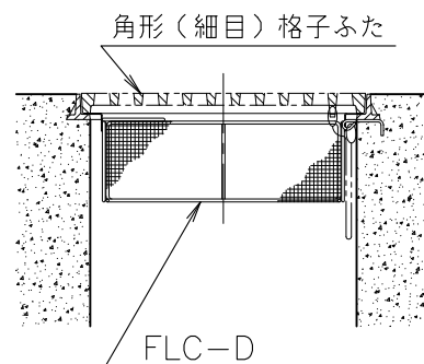
施工例(1:2)
