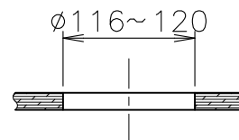
トラップ取付穴寸法
