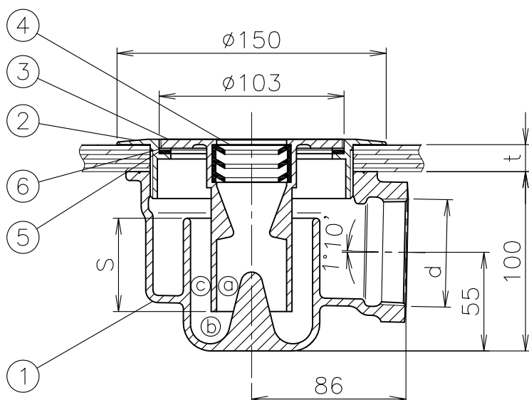
板厚と封水
