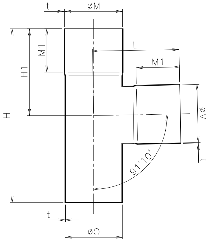
寸法表
