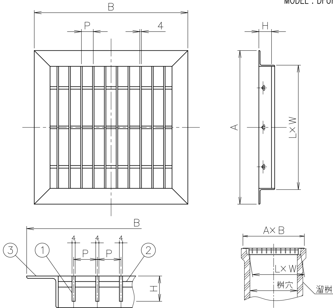
寸法表
