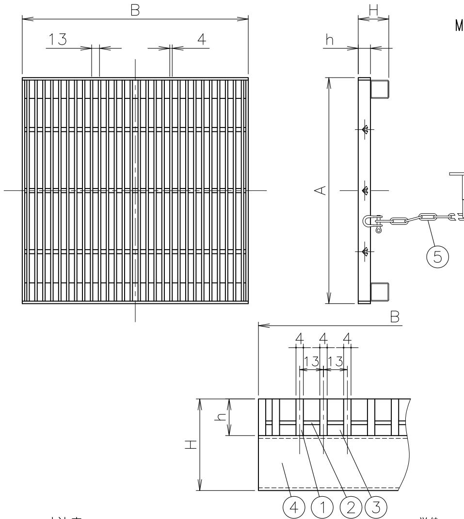
寸法表
