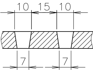
開口部詳細
