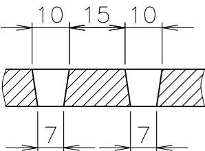
開口部詳細
