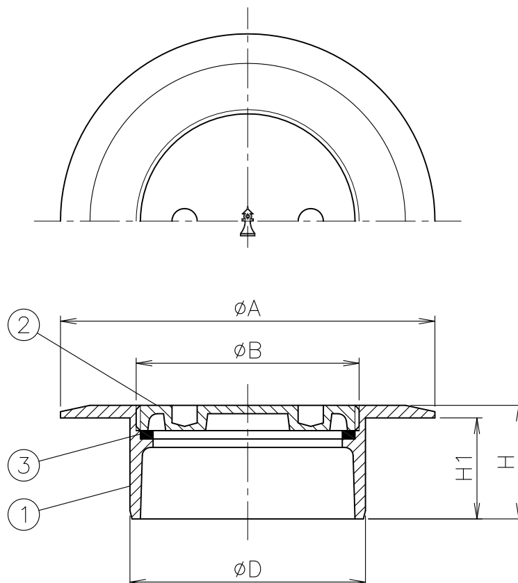
寸法表
