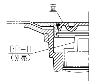
BP-H (プラグ) 取付図
