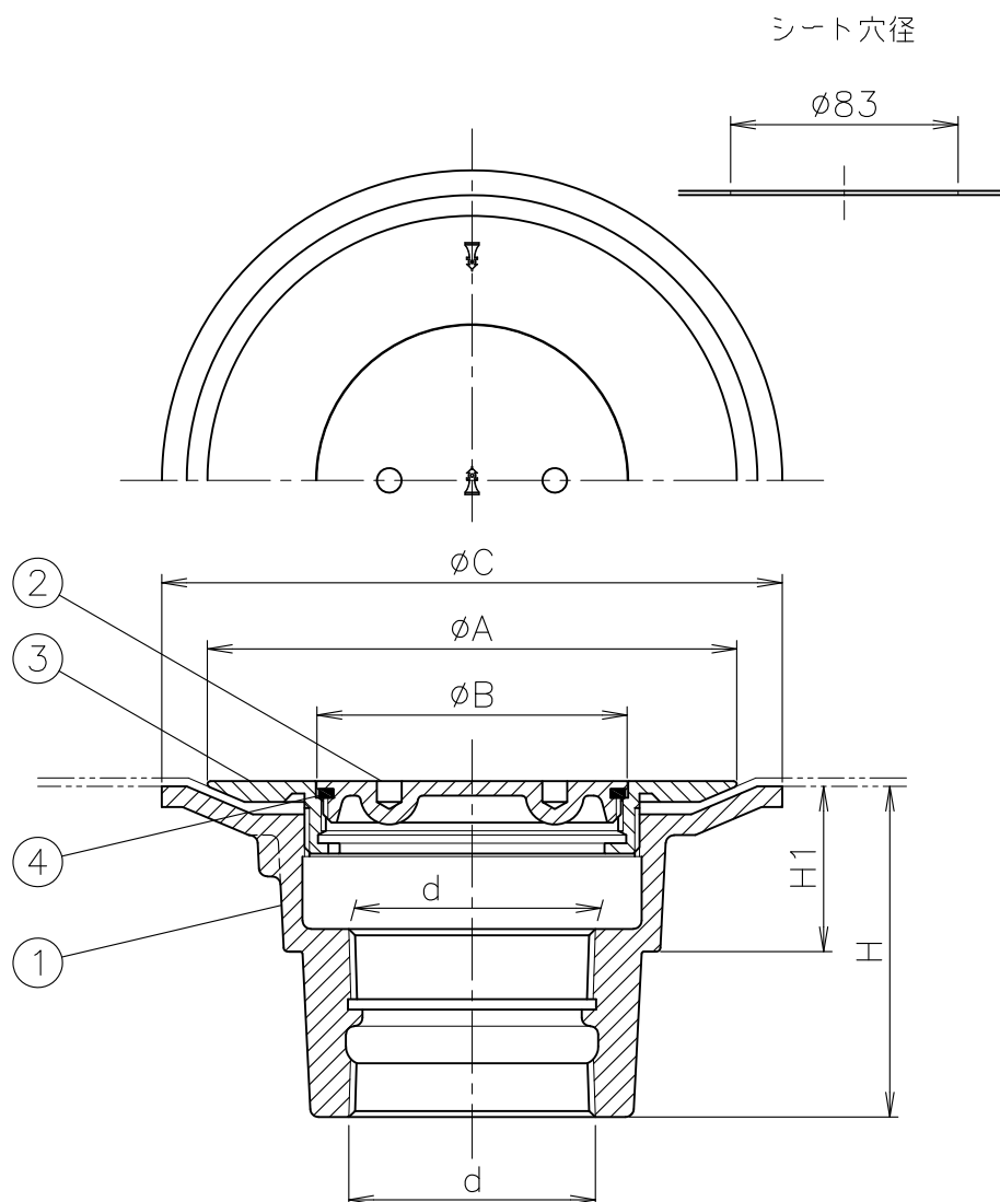
BP-H (プラグ) 取付図
