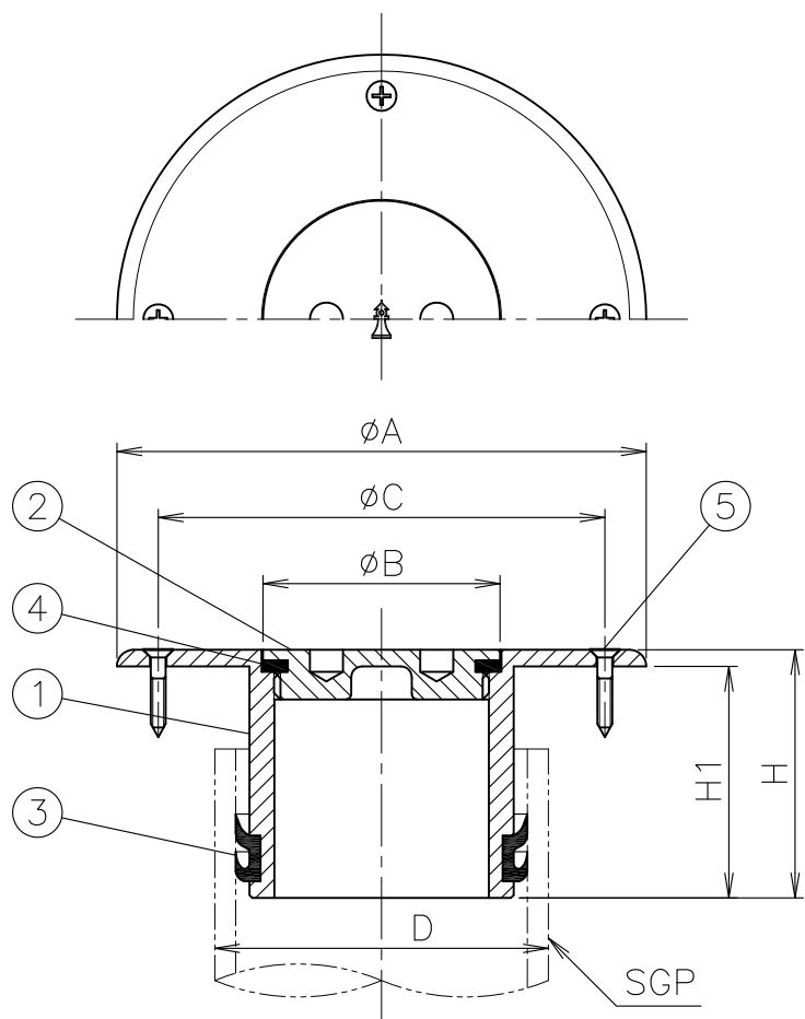
寸法表
